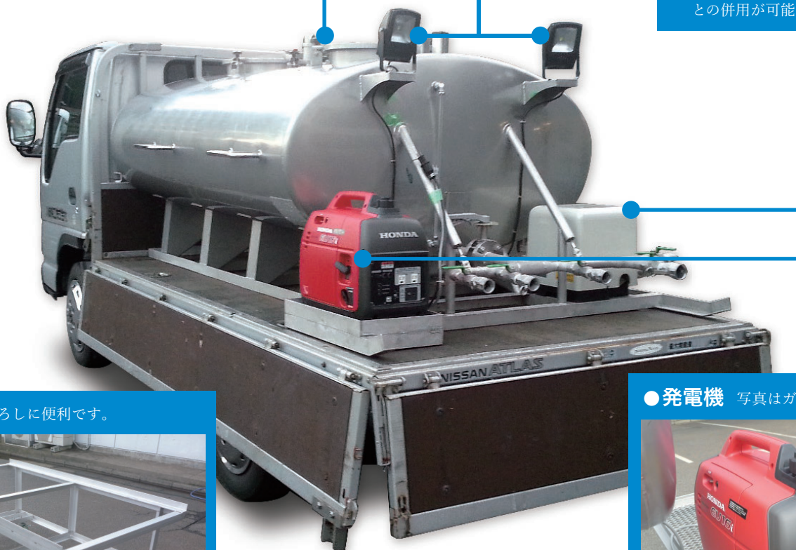
●電動ポンプ 加圧ポンプ搭載の場合は圧送給水との併用が可能です。
